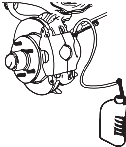
Рисунок 5 – Прокачка гидравлической тормозной системы
