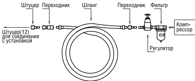
Рисунок 3 – Схема подключения к компрессорной установке
