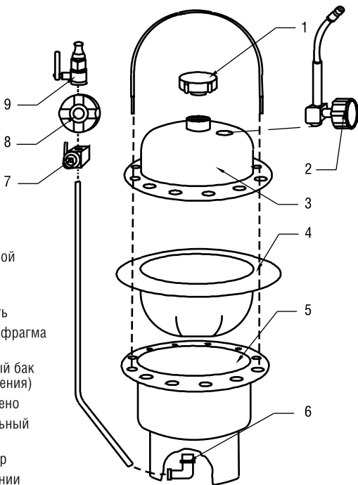
Рисунок 2 – Устройство изделия
